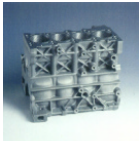
Zylinderkurbelgehäuse ( lost foam, Prototyp )
