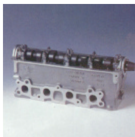
Zylinderkopf 4 Zylinder Diesel, ZSB
